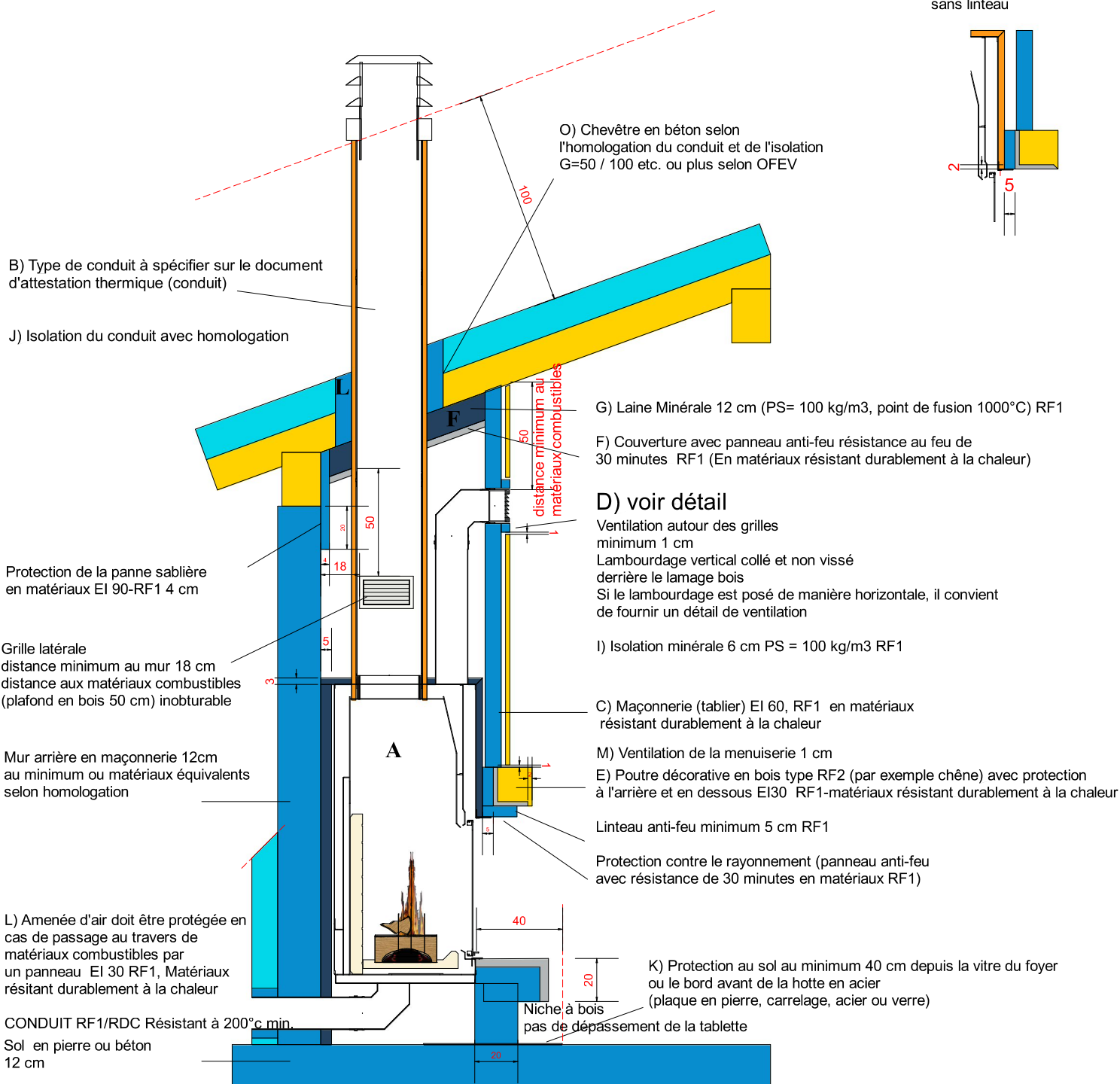
E) Variante poutre sans linteau
